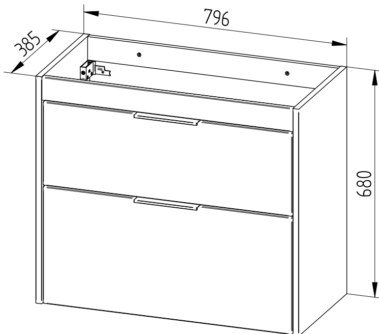
TYP 03
