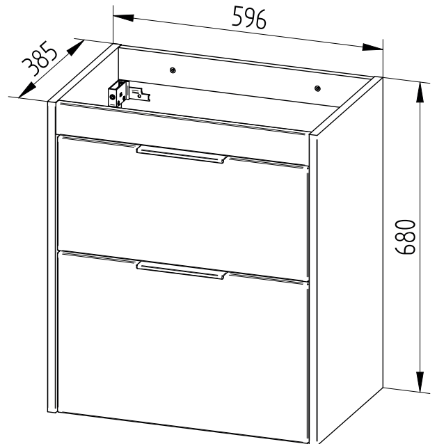
TYP 02
